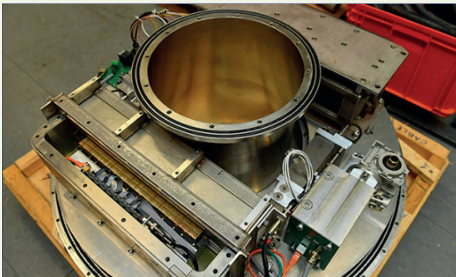
Внутреннее устройство инструмента ПГЭТ, который используется для проверки отработавшего ядерного топлива. (Фото: Д. Кальма/МАГАТЭ)
