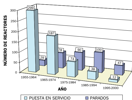
Figura 2. Histograma de doble columna que muestra el número decreciente de reactores de investigación que se pusieron en servicio y el número creciente que se llevaron a régimen de parada en cada decenio entre 1955 y 1994, y en los cinco años transcurridos de 1995 a 2000
