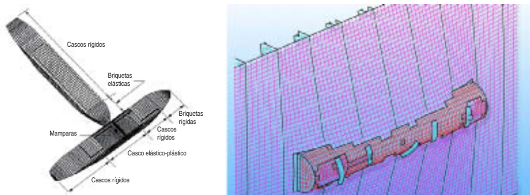
FIG. 1. Los modelos de colisiones de buques (izquierda) han indicado que la magnitud de las fuerzas de aplastamiento a las que probablemente estén sometidos los bultos de materiales radiactivos transportados por mar incluso en las colisiones más graves entre dos buques se ve limitada por la fuerza de la estructura lateral de la embarcación de transporte. El gráfico a la derecha muestra la salida del contenedor no dañado por el costado de un buque..
