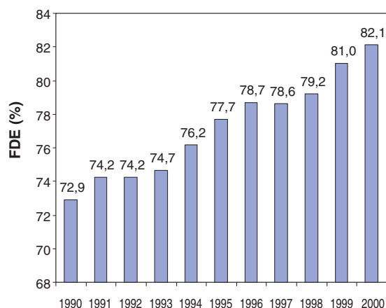
FIG. 1. Factor de disponibilidad de energía (FDE) medio mundial.
