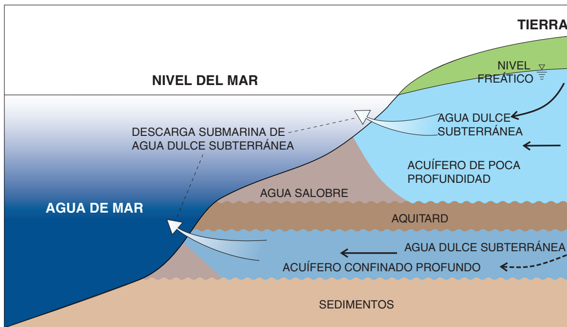
FIG. 3. Representación esquemática del proceso submarino de descarga de las aguas subterráneas.
